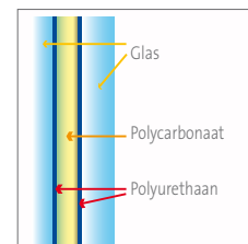
▲ Glas en Polycarbonaat inbraakvertragend
